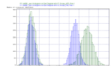
Figura 1.6 Istogrammi Frequenze Livelli (Q = 7) - Confronto PIN (SX) vs APD (DX)
