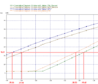
Figura 1.3 Q vs P 0 (dBm) - Confronto Ricevitori (4 casi - cfr. Tabella Comparativa 1.2)
